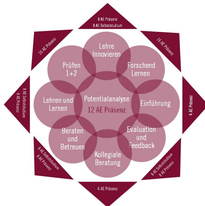
Abb. 2. Programmstruktur Basisbereich
